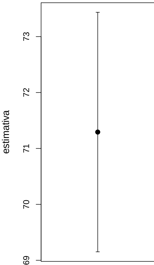
desvio-padrão dos tracos latentes
