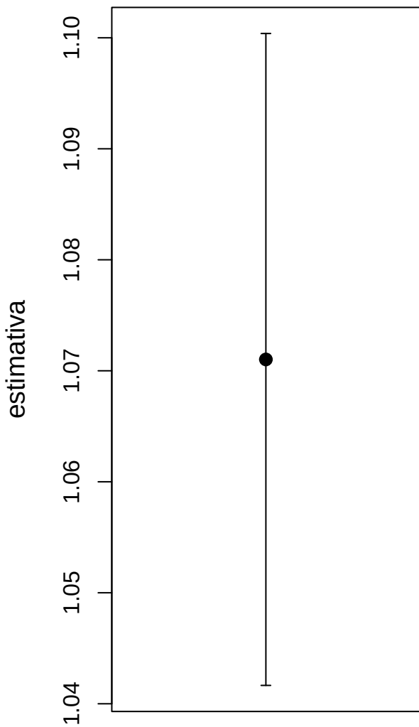
media dos tracos latentes
