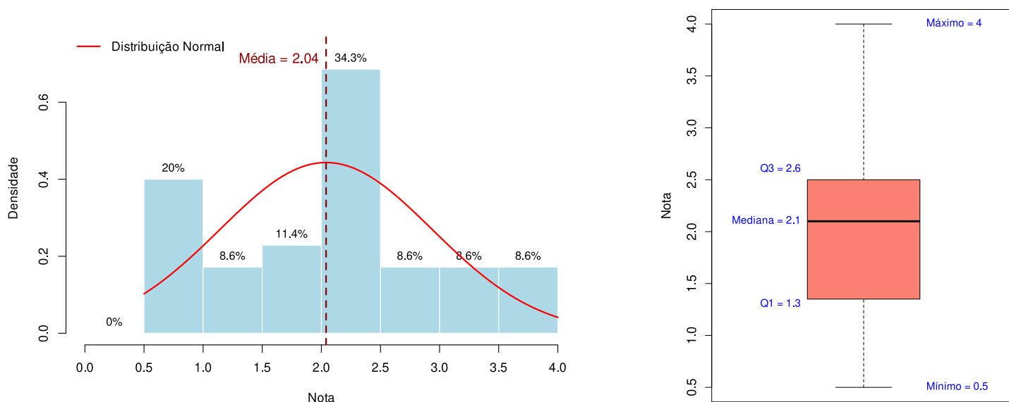
Figura 1: Histograma e boxplot da nota.
