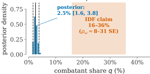
B. Posterior on q vs. IDF claim band
