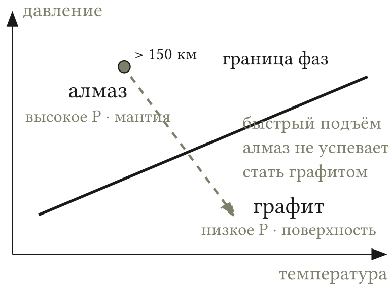
Рис. 1. На Р–Т диаграмме алмаз устойчив при высоком давлении (мантия, глубже 150 км), графит — у поверхности. Быстрый подъём кимберлита не даёт алмазу графитизироваться.
