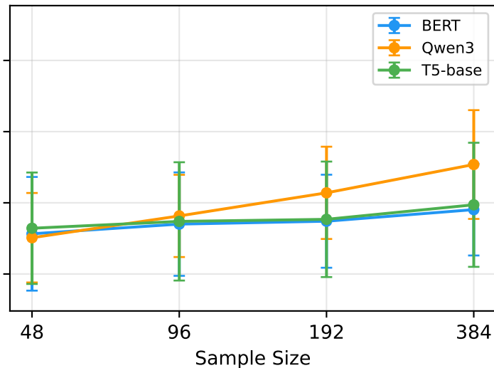
BitFit
