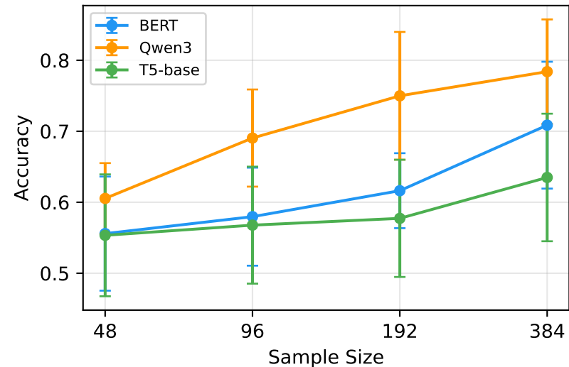
LoRA
