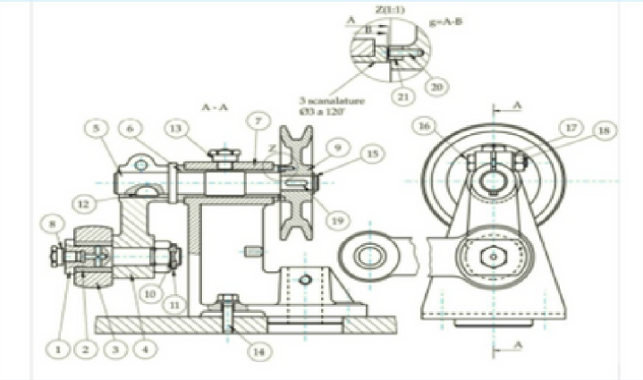
SCHEMA MECCANICO
