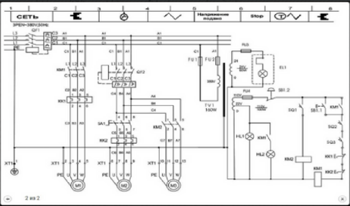
SCHEMA ELETTRICO
