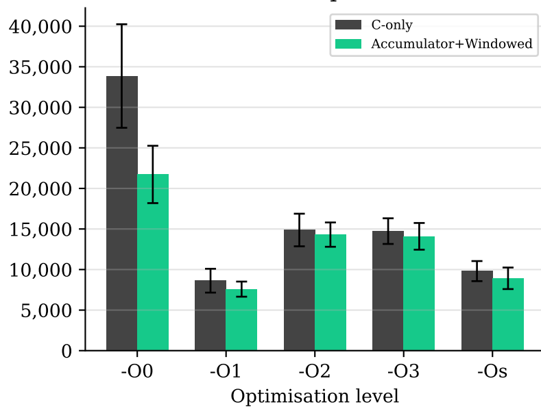
Encaps
