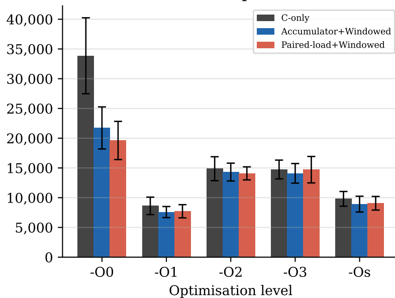
Encaps
