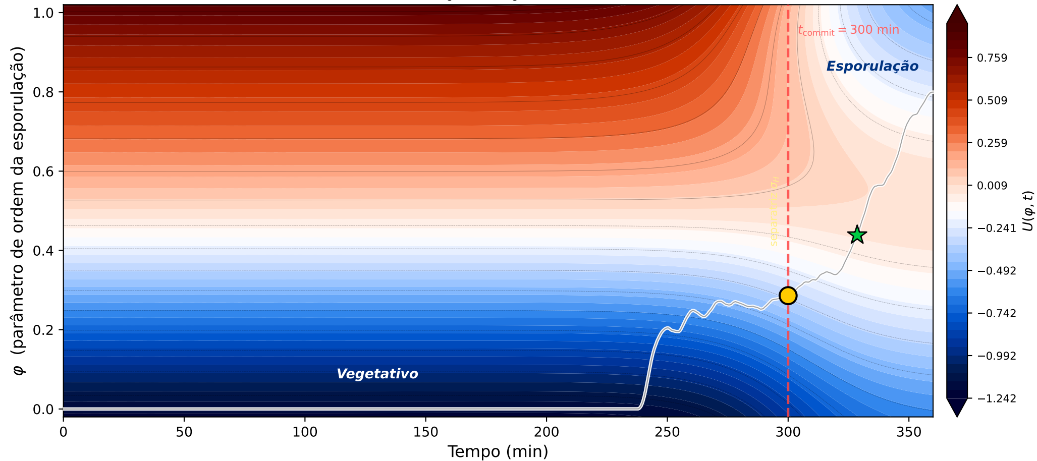
Paisagem de Potencial Epigenético – B. subtilis Esporulação Poço duplo analítico U(\varphi, t) = a\phi_c^4 - b(t)\phi_c^2 + c(t)\phi_c \cdot \varphi(t) médio de 50 réplicas
