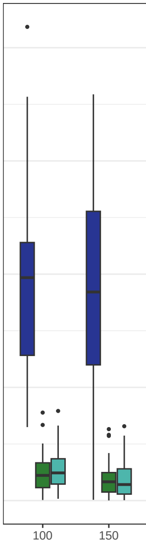
Noisy Variables
