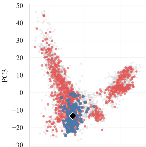
PEVmean-GA
