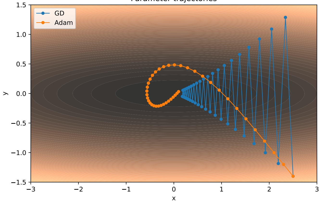
Parameter trajectories
