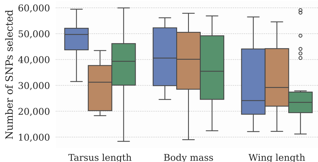
(d) SNPs selected by phenotype
