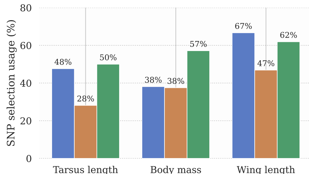
(d) SNPs selected by phenotype
