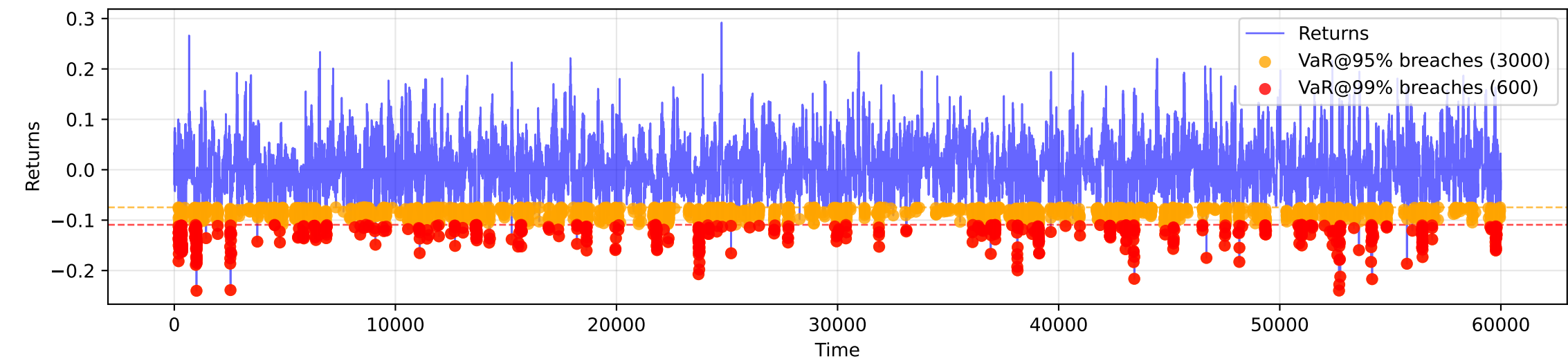
Ilm VaR Exceedances
