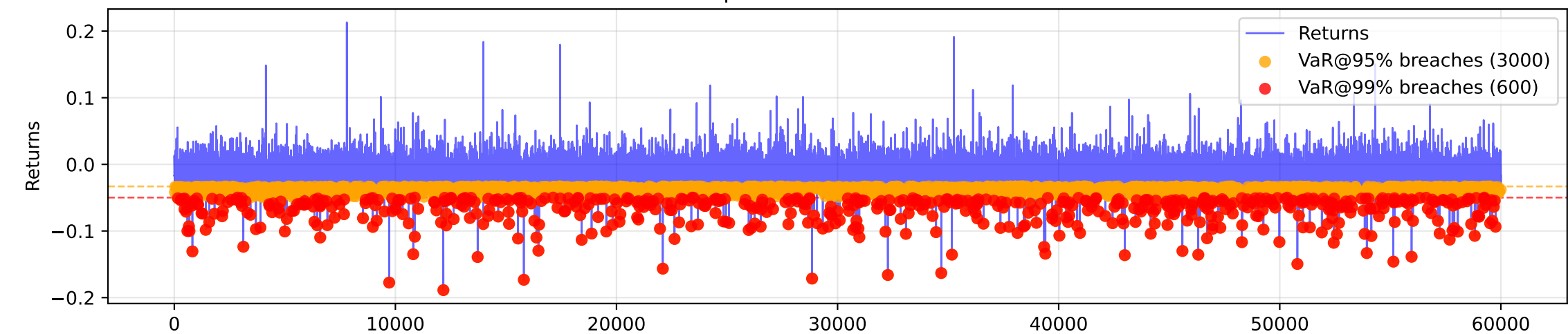
Ilm VaR Exceedances
