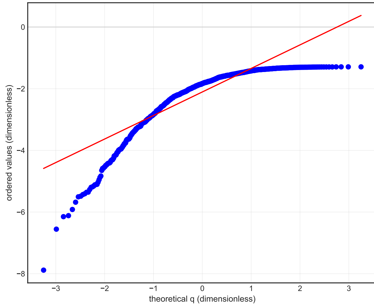
Q-Q left tail
