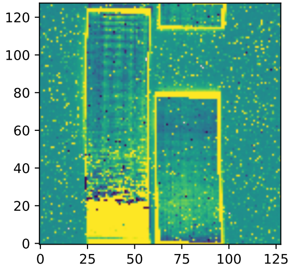
12um Zodi: 23.5 MJy/sr
