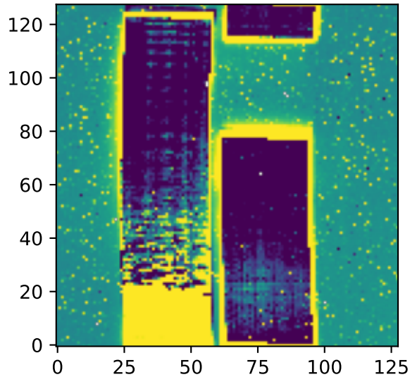
12um Zodi: 42.0 MJy/sr
