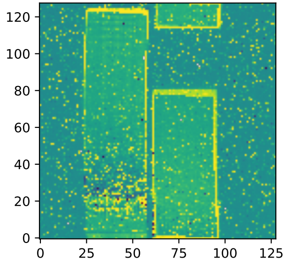
12um Zodi: 14.8 MJy/sr
