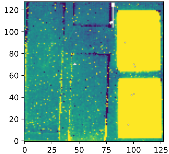
12um Zodi: 14.2 MJy/sr
