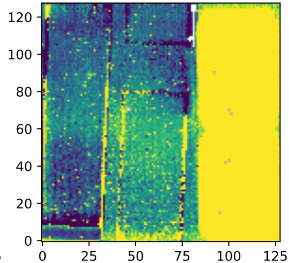
12um Zodi: 29.9 MJy/sr
