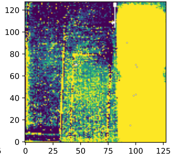
12um Zodi: 39.7 MJy/sr
