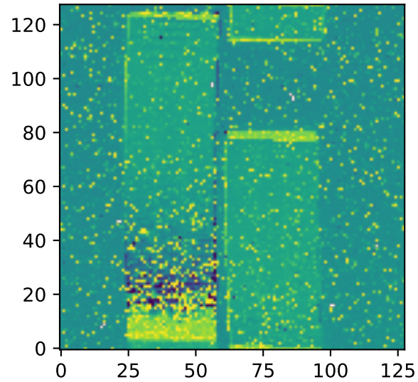
12um Zodi: 14.1 MJy/sr
