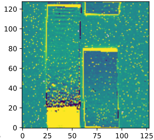
12um Zodi: 22.7 MJy/sr
