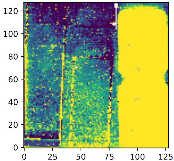
12um Zodi: 31.5 MJy/sr
