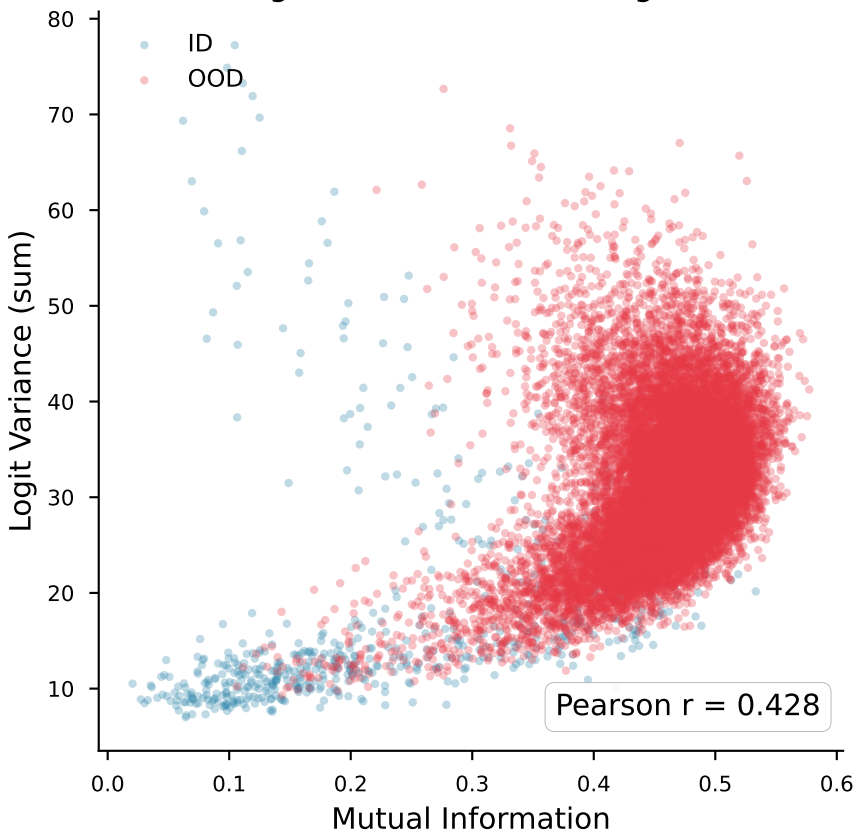
MI vs Logit Variance — ID vs organamnist
