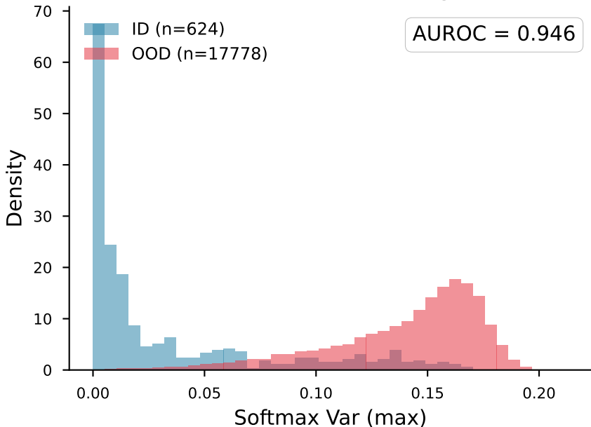
Softmax Var (max) — ID vs organamnist
