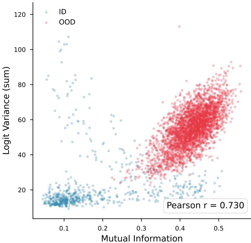
MI vs Logit Variance — ID vs bloodmnist
