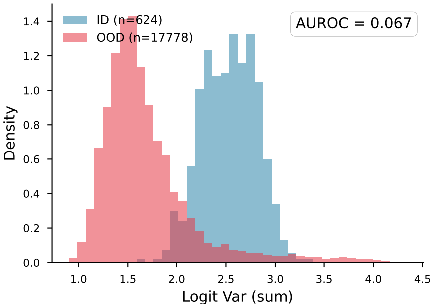
Logit Var (sum) — ID vs organamnist
