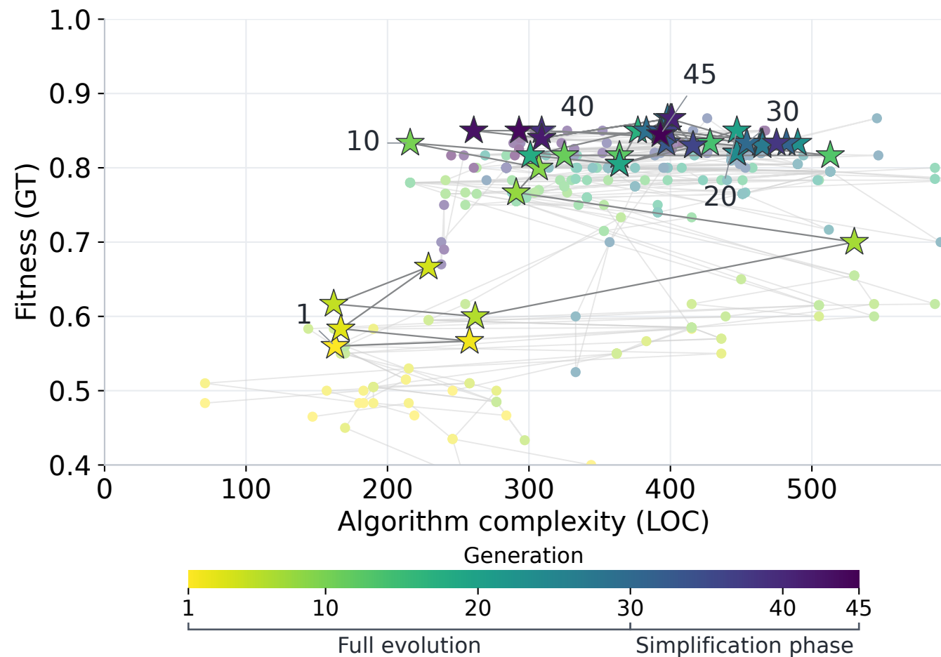
PySR evolution
