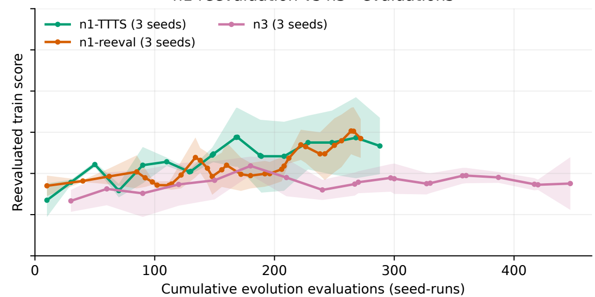
n1 reevaluation vs n3 · evaluations
