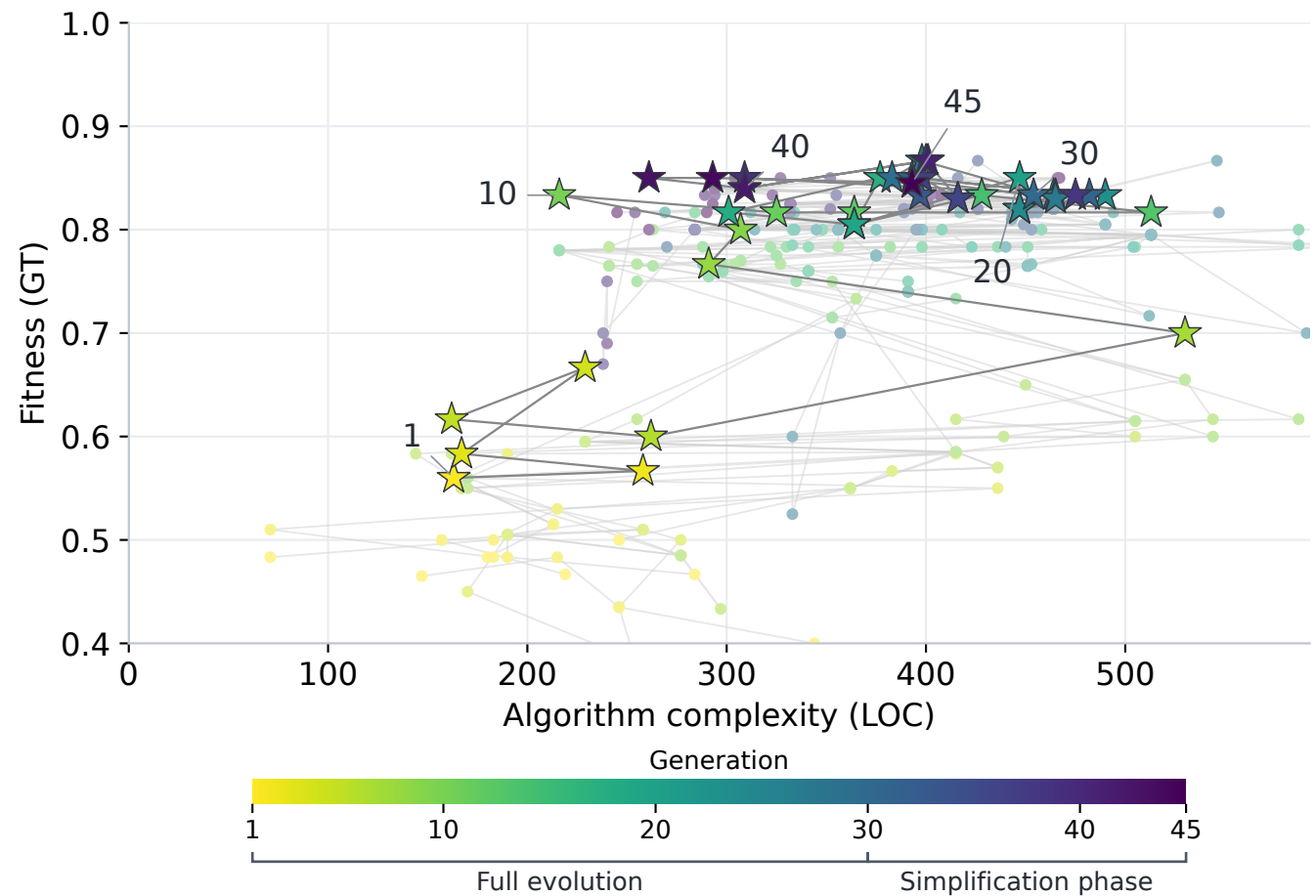
PySR evolution
