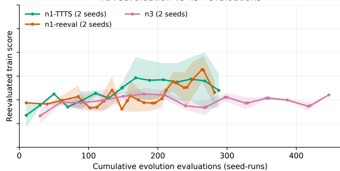
n1 reevaluation vs n3 · evaluations
