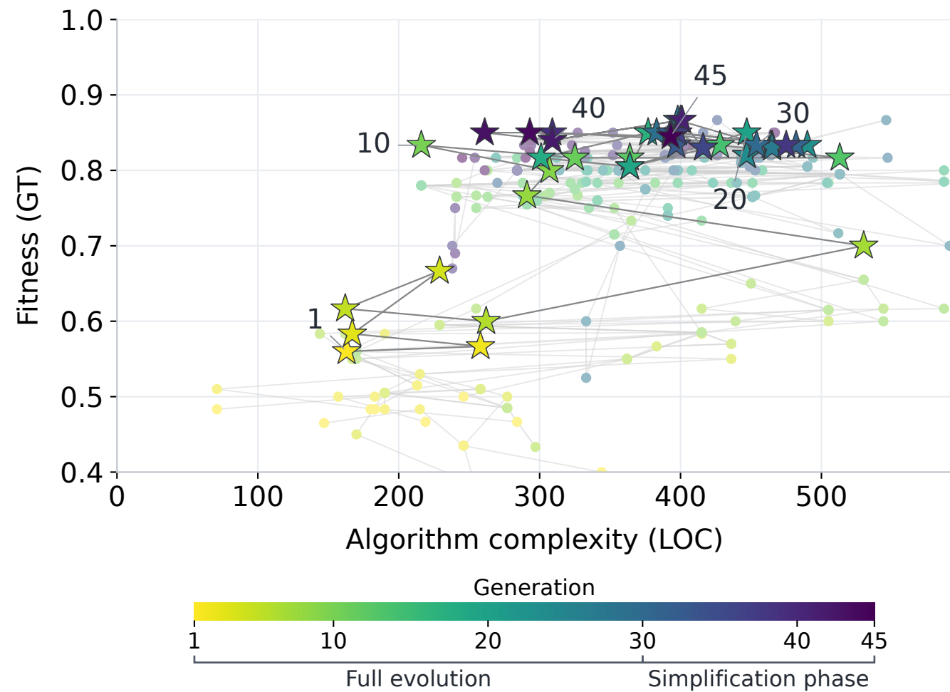
PySR evolution
