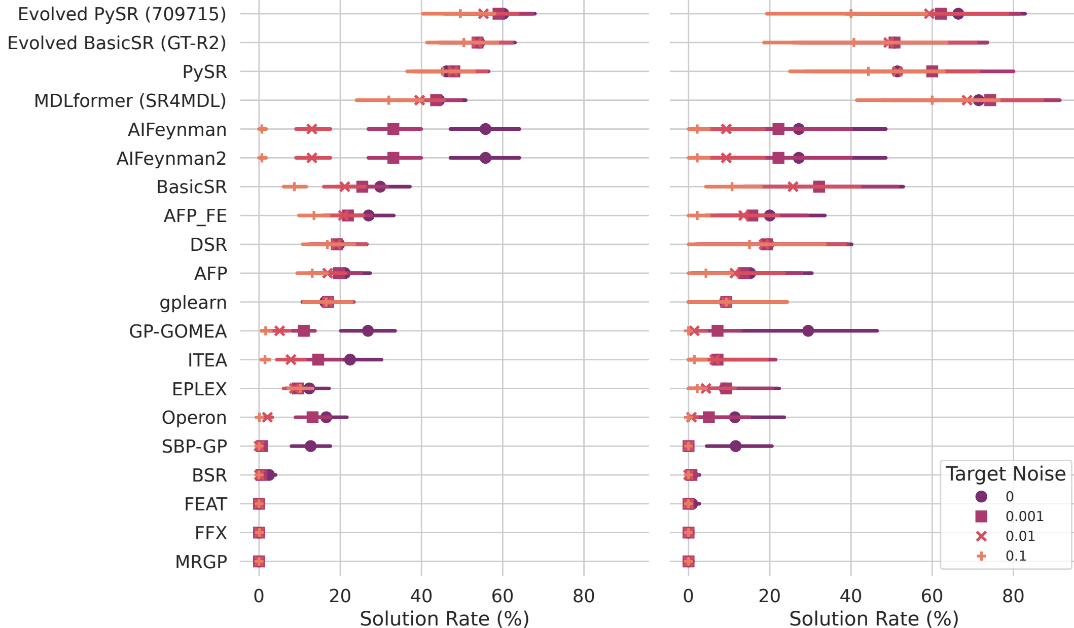
Feynman
