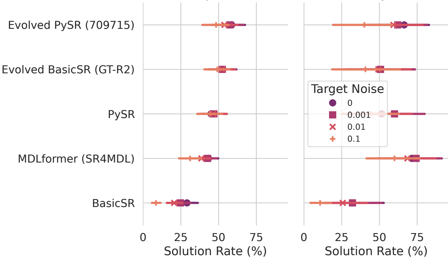
Feynman
