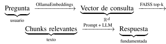
Figura 2. Pipeline de inferencia RAG.
