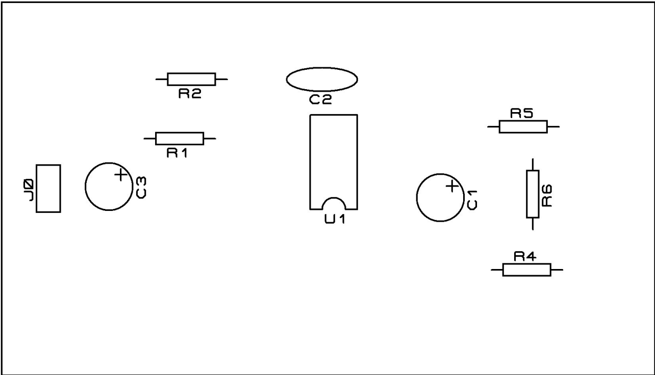
figure 6 : schéma d’implantation du dessus de la « carte lumière » du « système sonore et lumineux » (sans effet miroir)
