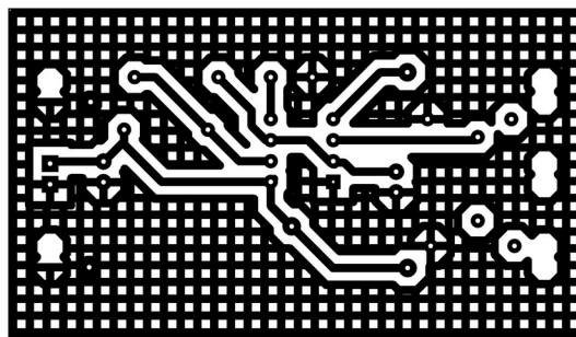
figure 4 : typon bottom de la « carte lumière » du « système sonore et lumineux » (sans effet miroir)
