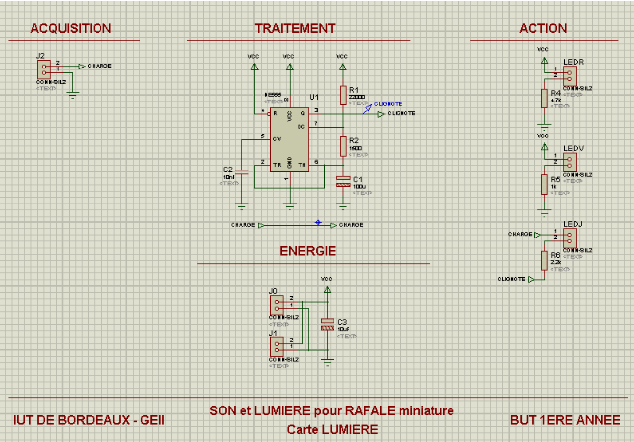
figure 1 : schéma électrique de la « carte lumière » du « système sonore et lumineux »
