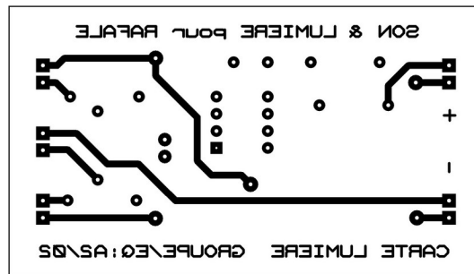
figure 3 : typon top de la « carte lumière » du « système sonore et lumineux » (avec effet miroir)
