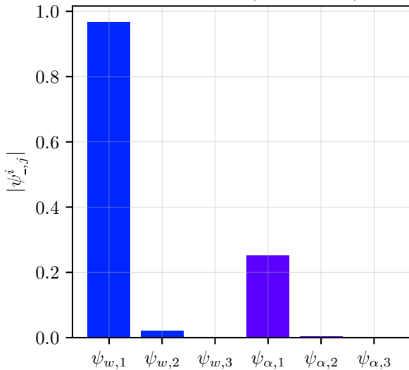
Mode 1 : \psi^1 (f=1.95 Hz)
