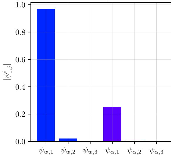
Mode 1 : \psi^1 (f=1.95 Hz)
