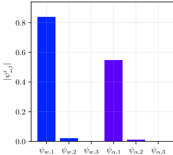
Mode 1 : \psi^1 (f=1.93 Hz)
