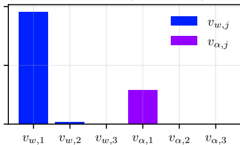
Mode 2 : v^2 (f=8.47 Hz)
