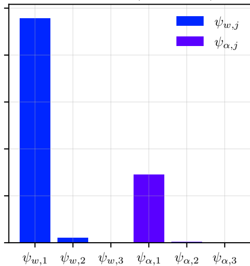
Mode 2 : \psi^2 (f=8.47 Hz)
