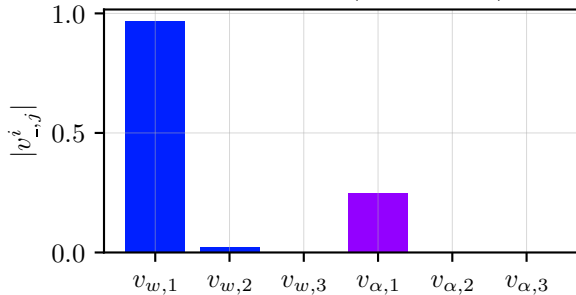
Mode 1 : v^1 (f=1.95 Hz)
