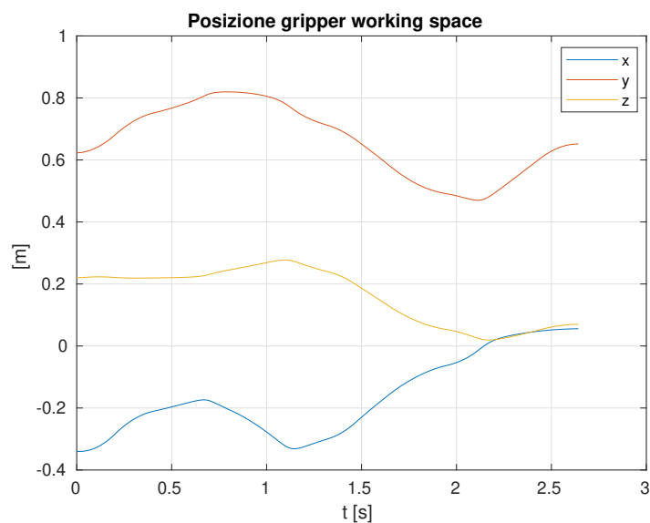
Figura 3.7: Posizioni assunte dal gripper nel working space nella traiettoria assegnata.
