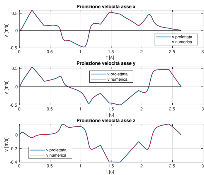
Figura 3.8: Velocità assunte dal gripper nel working space nella traiettoria assegnata.
