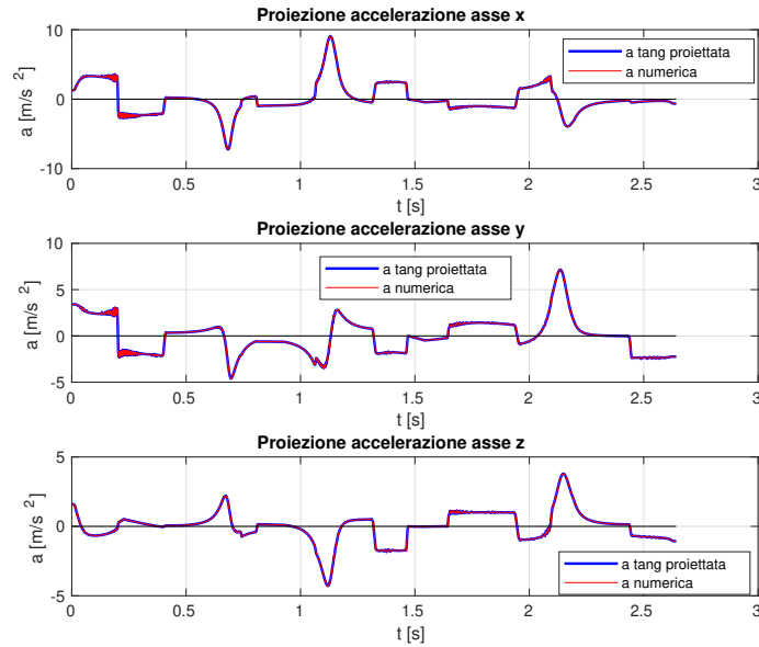
Figura 3.9: Accelerazioni assunte dal gripper nel working space nella traiettoria assegnata.
