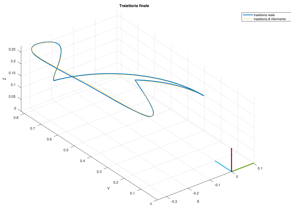
Figura 4.1: Confronto tra la traiettoria di riferimento e la traiettoria compiuta dal robot.
