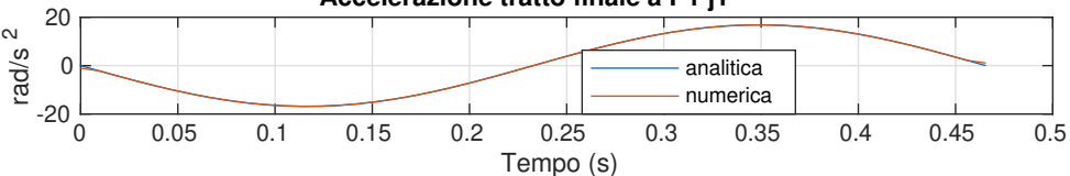
Accelerazione tratto finale a P1 j2
