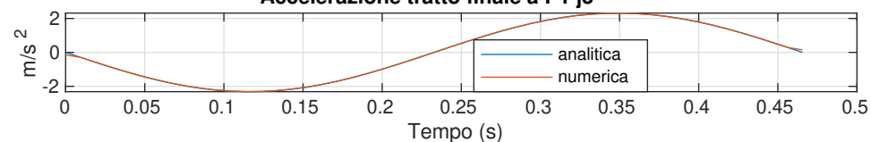
Accelerazione tratto finale a P1 j4
