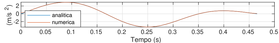
Accelerazione tratto finale a P1 asse y
