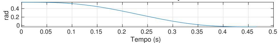
Traiettoria tratto finale a P1 j2
