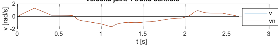
Velocità joint 4 tratto centrale
