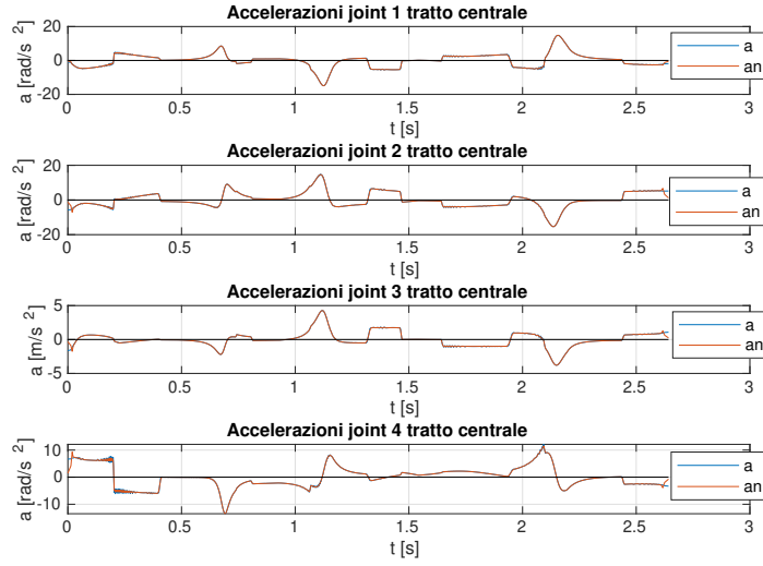
Figura 3.11: Accelerazioni dei giunti nella traiettoria assegnata.
