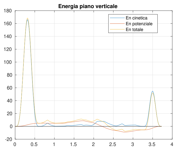
Figura 3.18: Energia durante la simulazione.
