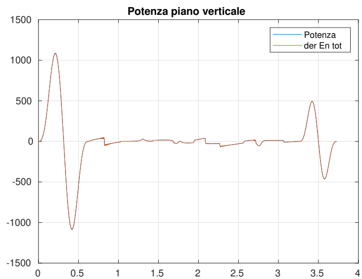
Figura 3.19: Potenza assorbita dai giunti durante la simulazione.
