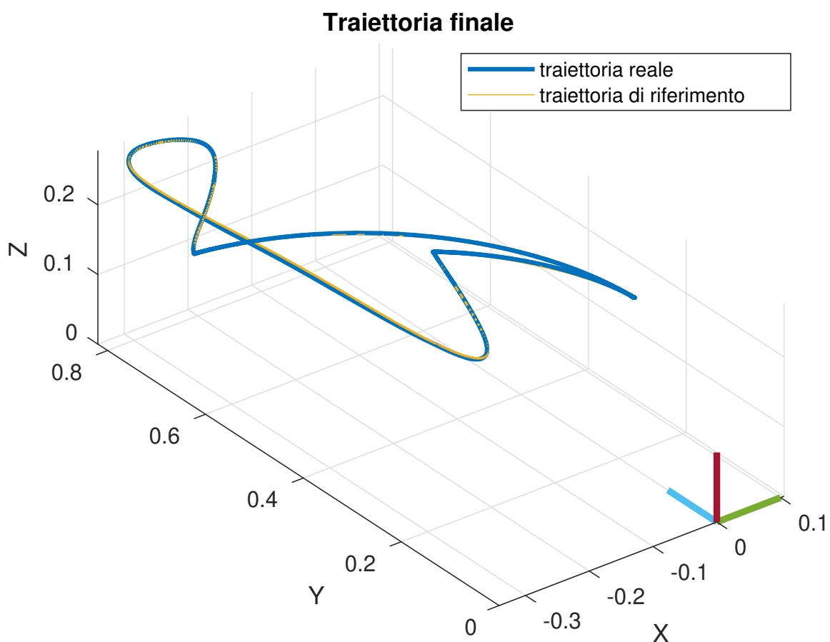
Figura 4.1: Confronto tra la traiettoria di riferimento e la traiettoria compiuta dal robot.
