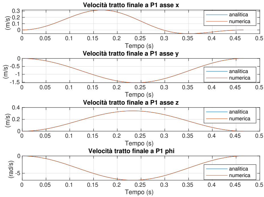
Figura 3.8: Velocità del tratto finale.
