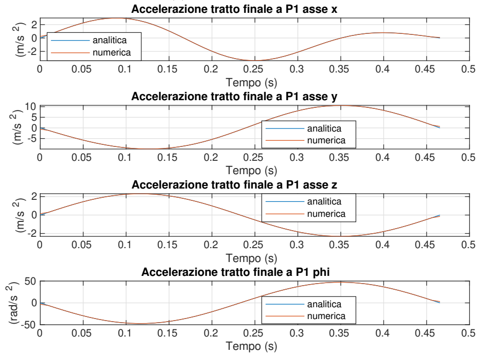
Figura 3.9: Accelerazione del tratto finale.
