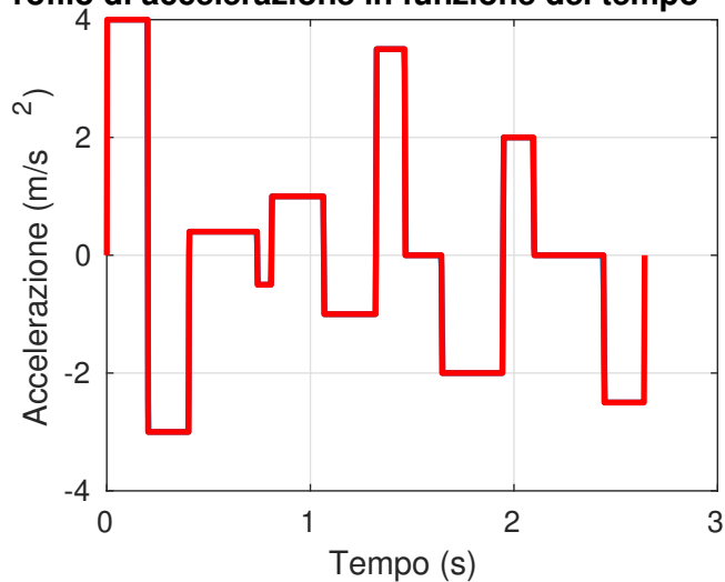
Profilo di accelerazione in funzione del tempo
