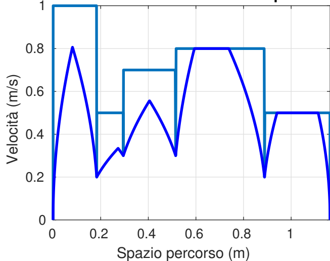
Profilo di velocità in funzione dello spazio
