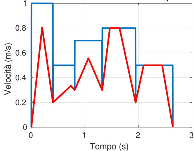
Profilo di velocità in funzione del tempo
