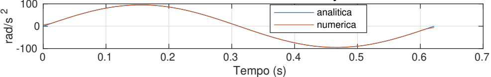
Accelerazione tratto iniziale da P1 j4
