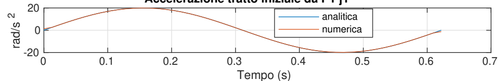
Accelerazione tratto iniziale da P1 j2
