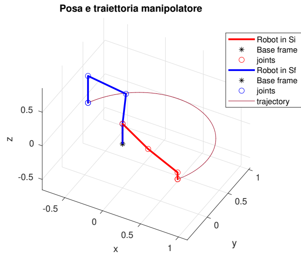
Figura 2.1: Posa e traiettoria compiuta dal manipolatore nella simulazione con traiettoria curvilinea.
