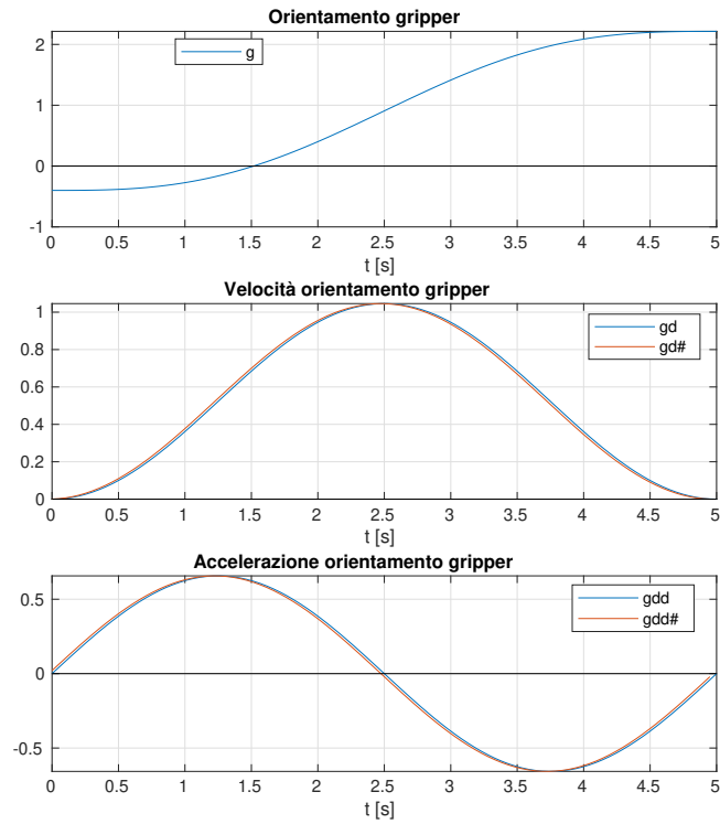
Figura 2.5: Coordinate di orientamento, velocità ed accelerazione del quarto giunto rotoidale (gripper). Le grandezze che terminano con # sono state ricavate tramite derivazione alle differenze finite delle rispettive velocità.
