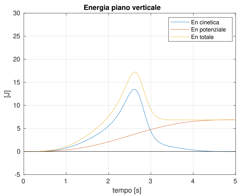
Figura 2.16: Energia assorbita dai giunti nella traiettoria simulata.
