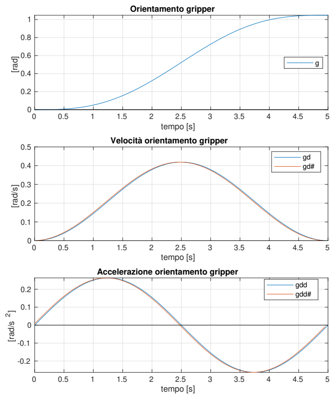
Figura 2.10: Orientamento del gripper nel sistema di riferimento alla base del robot.
