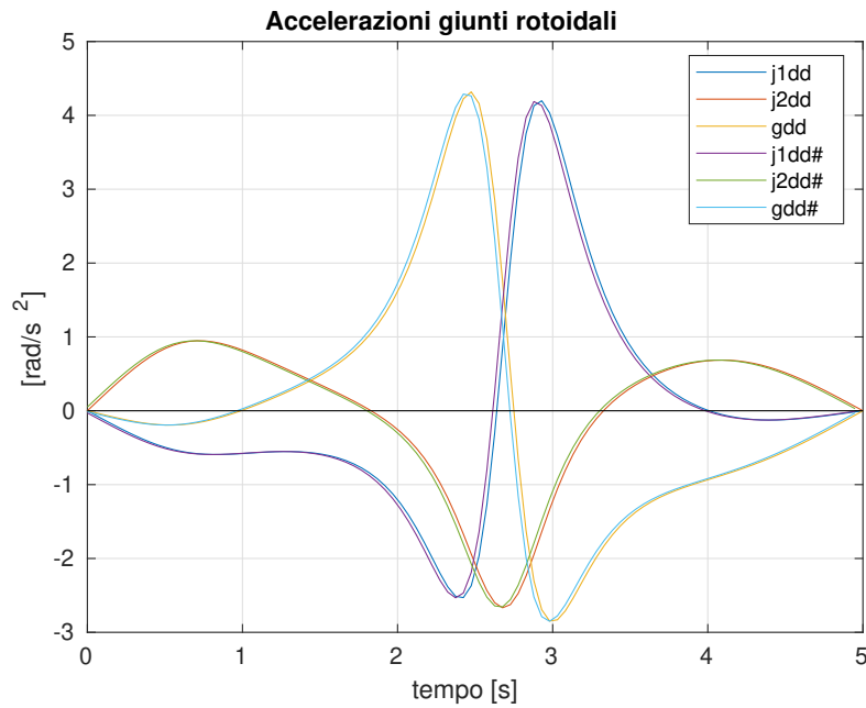
Figura 2.13: Accelerazione dei giunti durante la traiettoria simulata.
