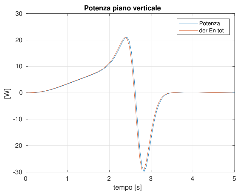
Figura 2.17: Potenza assorbita dai giunti nella traiettoria simulata.
