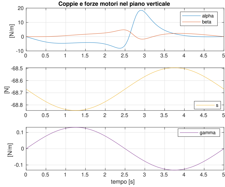
Figura 2.15: Coppie e forze della traiettoria simulata.
