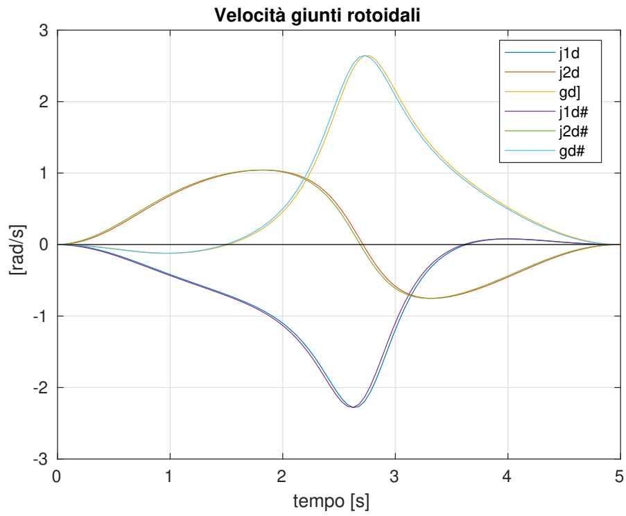
Figura 2.12: Velocità dei giunti durante la traiettoria simulata.
