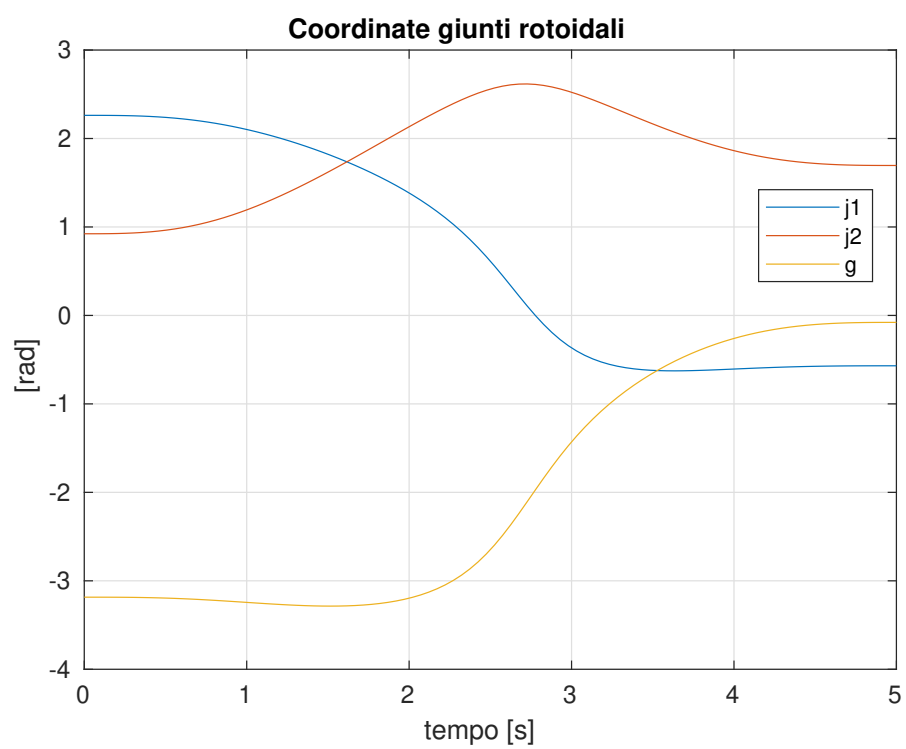
Figura 2.11: Orientamento dei giunti durante la traiettoria simulata.
