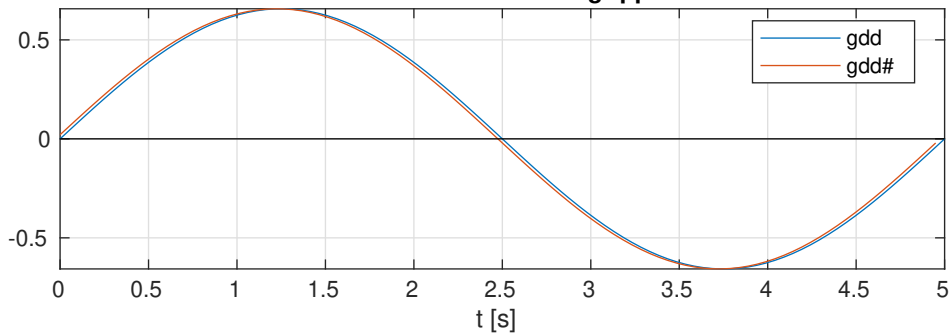
Accelerazione orientamento gripper
