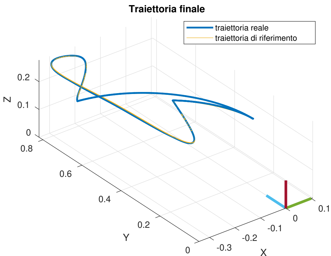
Figura 4.2: Confronto tra la traiettoria di riferimento e la traiettoria compiuta dal robot.
