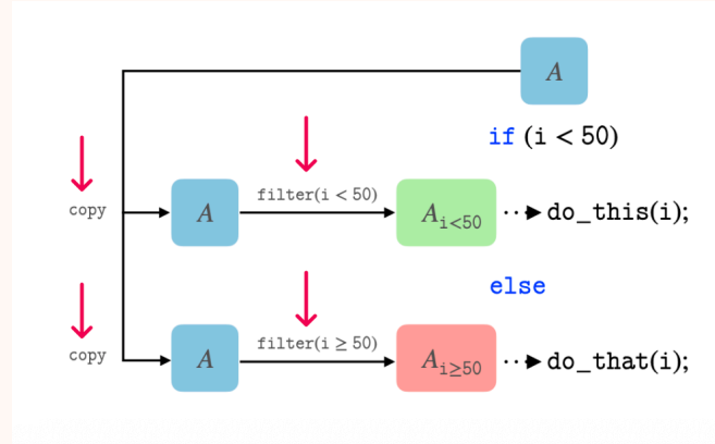
Figura 44: L'immagine illustra l'uso dell'operatore di filtro per gestire un ramo condizionale in un CFG. Lo stato astratto A viene filtrato in due stati distinti in base alla condizione c e alla sua negazione \neg c .
